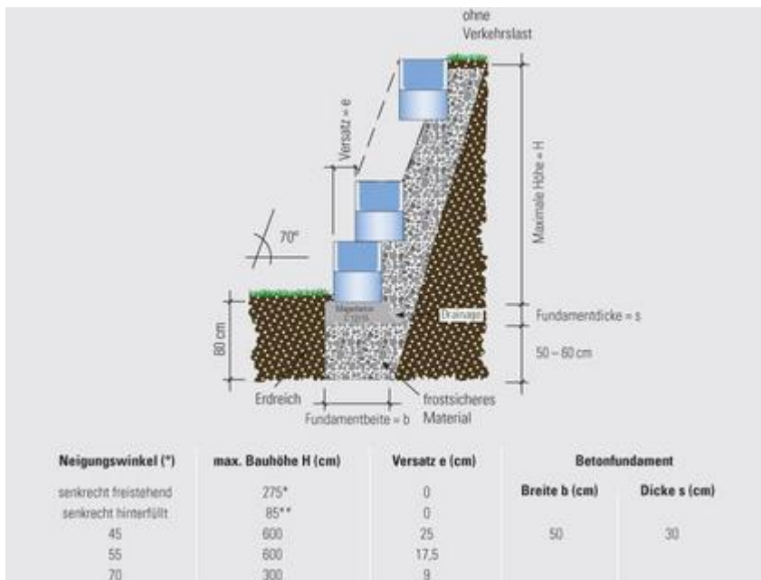
Böschungsbefestigung mit 70°-Neigung
