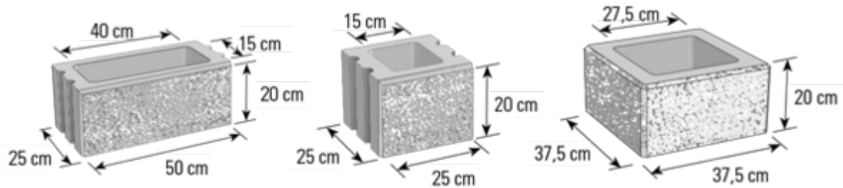
Grundelement
