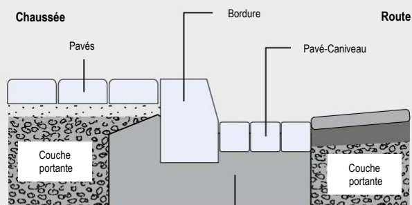
Exemple de réalisation d'un caniveau 3 files de pavés, largeur env. 50 cm
