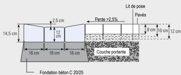
Exemple de réalisation du Forme-Caniveau
