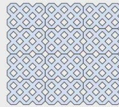
Dimension modulaire (cm) avec 40% de cavités 60,8/40,8
