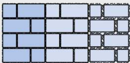
Pose combinée MultiTec, MultiTec-Aqua et MultiTec-Éco
