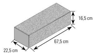
Typ 1: Grundelement groß Sichtflächen feingestrahelt, Köpfe un- bearbeitet, Oberseite feingestrahelt
