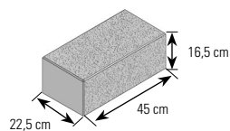
Typ 2: Grundelement klein Sichtflächen feingestrahelt, Köpfe un- bearbeitet, Oberseite feingestrahelt
