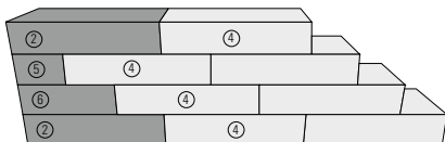
Aufbau Mauerkopf im getreppten Drittversatz
