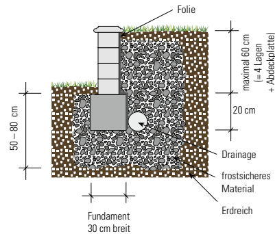
Senkrechter Aufbau, hinterfüllt, ohne Verkehrsast
