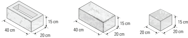
Grundelement
