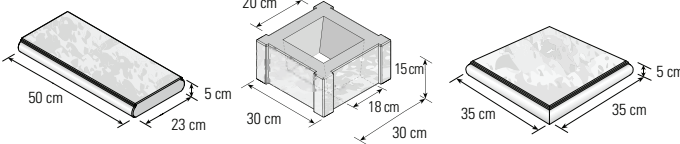
Mauer-Abdeckplatte
