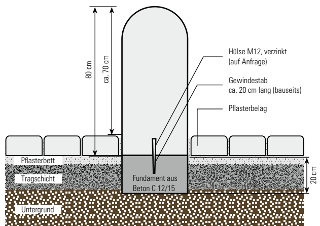
Einbaubeispiel MultiKegelpoller
