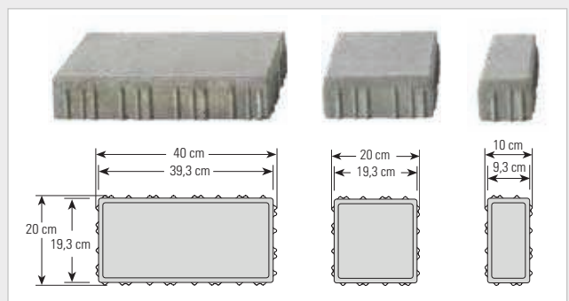
kombinierte Verlegung aus MultiTec, MultiTec-Aqua und MultiTec-Öko
