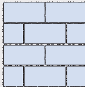
MultiTec-Aqua 40/20 Als Halbstein wird der MultiTec-Aqua 20/20 verwendet.
